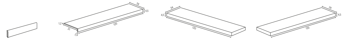
BATTISCOPA 7,5x60 cm - 3"x24" ± 10 mm NATURALE GRADINO PLUS BORDO 34x120x4,5 cm Rect - 13 3/8" x48"x1 3/4" ± 9,5 mm NATURALE GRADINO PLUS ANGOLARE DX 34x120x4,5 cm Rect - 13 3/8" x48"x1 3/4" ± 9,5 mm NATURALE GRADINO PLUS ANGOLARE SX 34x120x4,5 cm Rect - 13 3/8" x48"x1 3/4" ± 9,5 mm NATURALE
